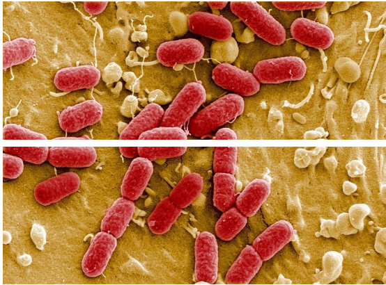
Escherichia Coli
